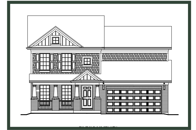
Elevation B
