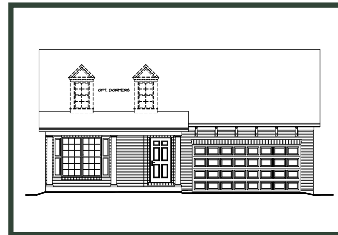
Elevation A
